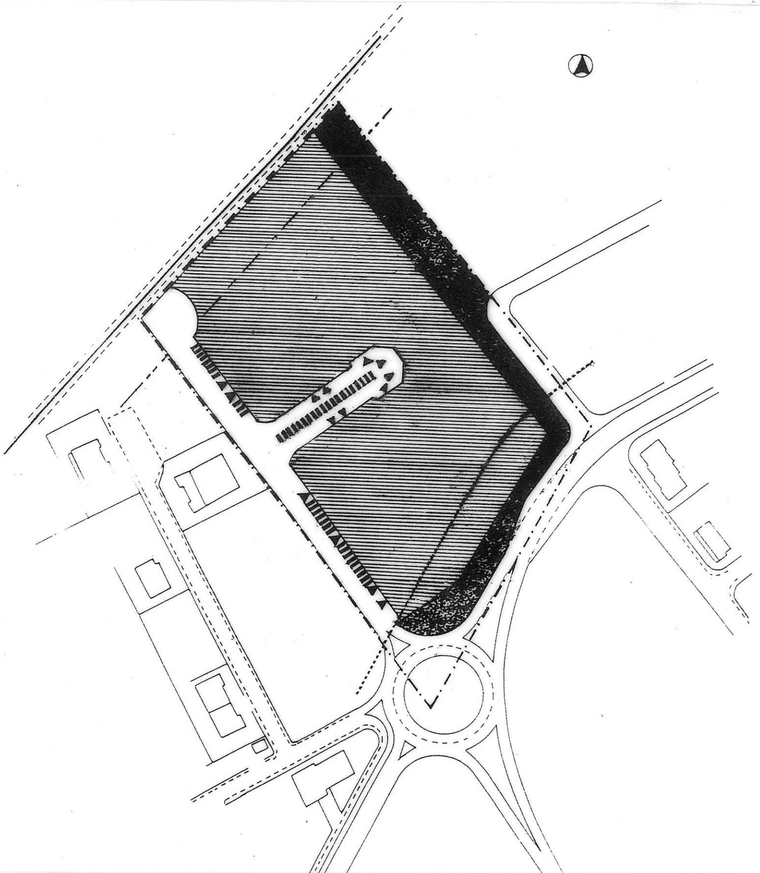
SCHEMA PLANIMETRICO - SCALA 1:2000 (prescrittivo)
